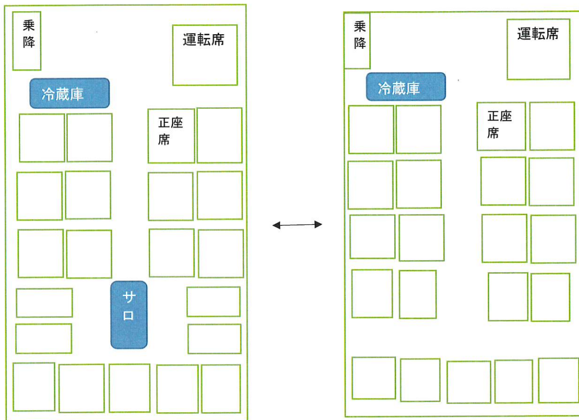
小型(サロン)バス 正座席21 回転サロン・2列シート サロン、冷蔵庫、、貫通式トランク
